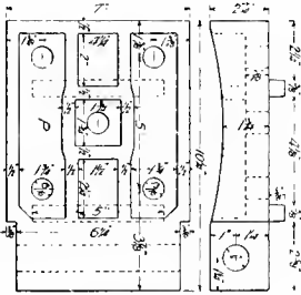
Figs. 5526-5527. STOP-PLATE.
